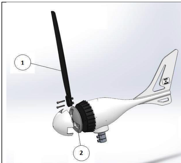
Рисунок 5 – Сборка ветрогенератора.
