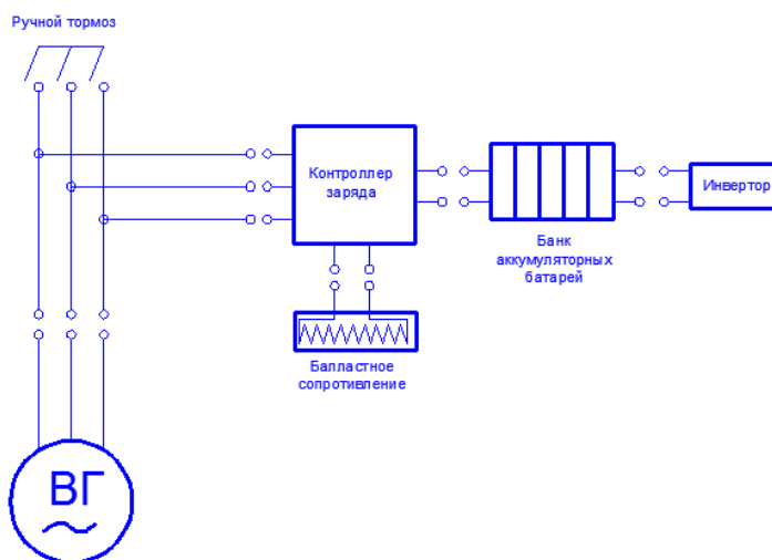
Рисунок 13 – Схема ручного торможения ветрогенератора.
