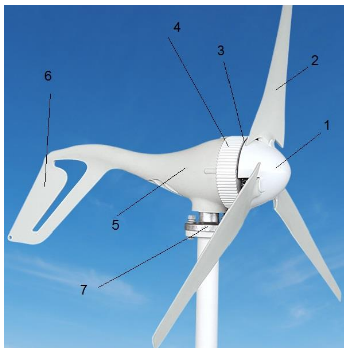
Рисунок 2 – Конструктивные элементы ветрогенератора.
